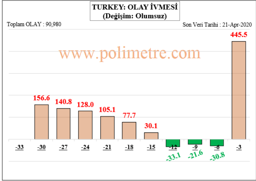
Şekil 3: Üç Günlük Fasıllarla OLAY İvmesi Değişimi – TÜRKİYE
