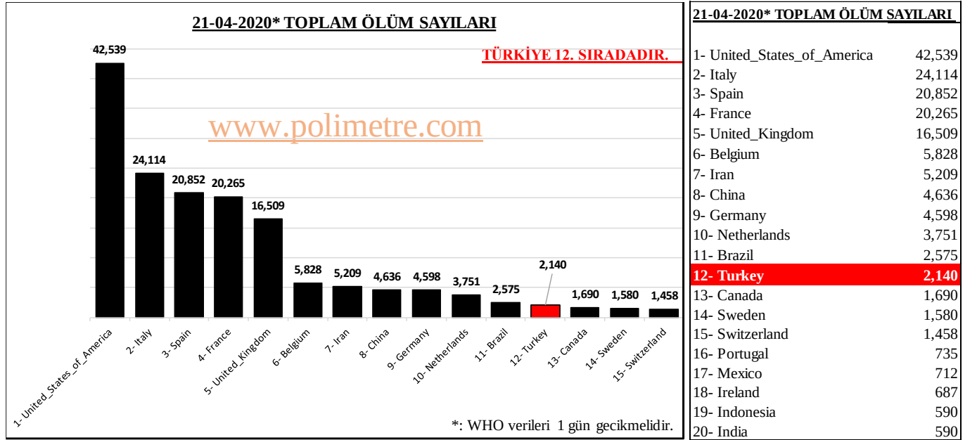
Şeki 8: Toplam ÖLÜM Sayıları En Yüksek Ülkeler ve ÖLÜM Sayıları
