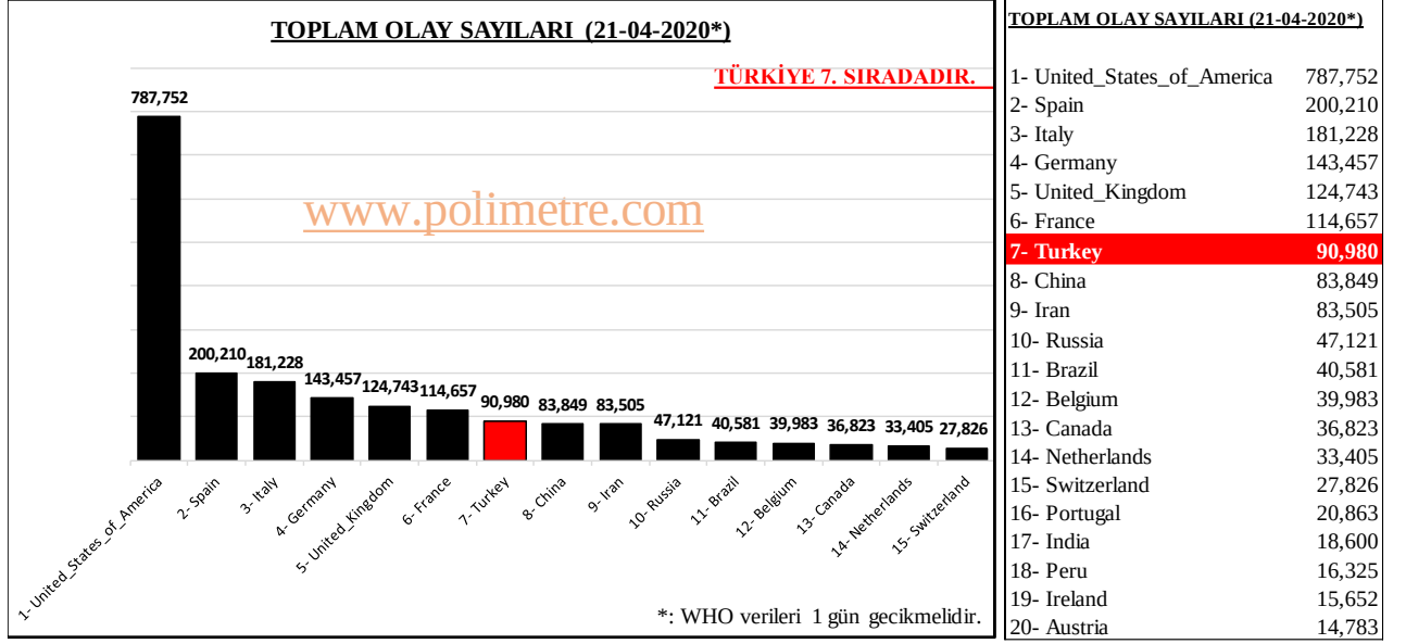
Şeki 7: Toplam OLAY Sayıları En Yüksek Ülkeler ve OLAY Sayıları
