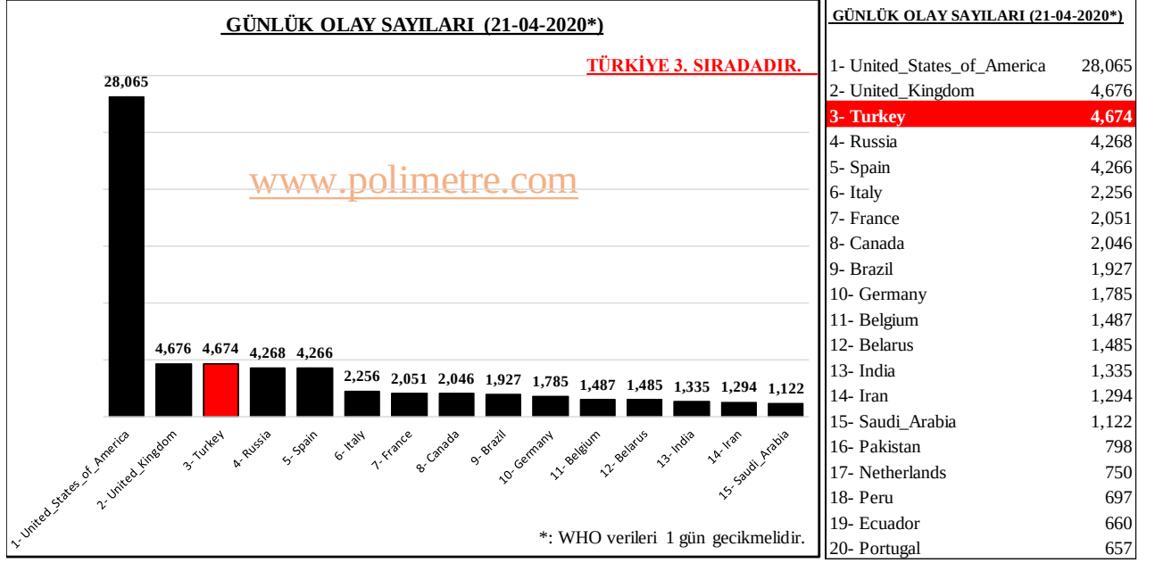
Şekil 5: Günlük OLAY Sayısı En Yüksek Ülkeler ve OLAY Sayıları
