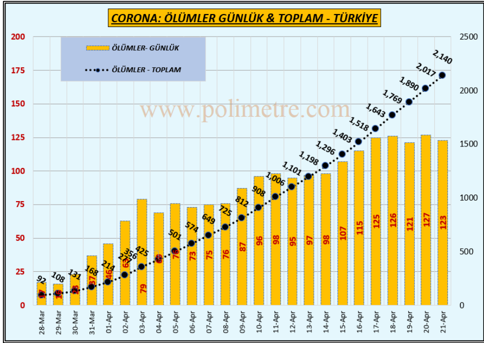
Şekil 2: Günlük ve Toplam ÖLÜM Sayıları – TÜRKİYE
