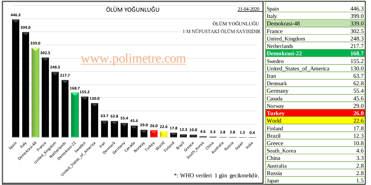
Şekil 10: Dünya’da, DEMOKRASİ-22, DEMOKRASİ-48 Ülkelerinde ve Diğer Bazı Ülkelerdeki ÖLÜM Yoğunlukları (1 Milyon Kişideki ÖLÜM Sayısıdır)
