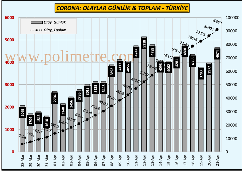
Şekil 1: Günlük ve Toplam OLAY Sayıları - TÜRKİYE
