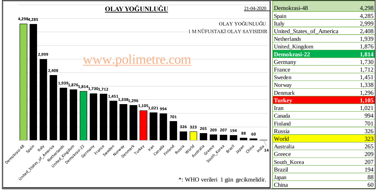
Şekil 9: Dünya’da, DEMOKRASİ-22 1 , DEMOKRASİ-48 2 Ülkelerinde ve Diğer Bazı Ülkelerdeki OLAY Yoğunlukları (1 Milyon Kişideki OLAY Sayısıdır)
