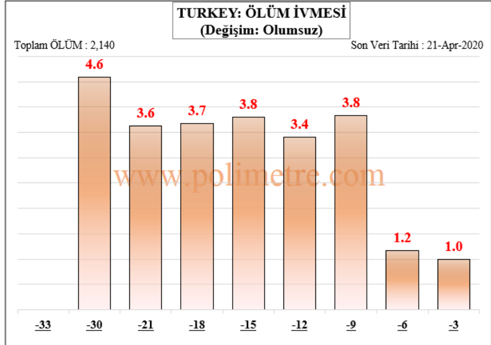
Şekil 4: Üç Günlük Fasıllarla ÖLÜM İvmesi Değişimi - TÜRKİYE
