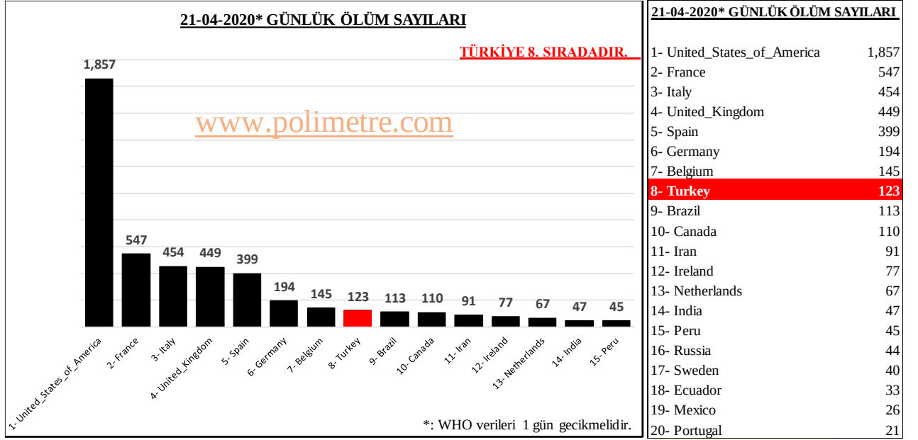
Şekil 6: Günlük ÖLÜM Sayısı En Yüksek Ülkeler ve ÖLÜM Sayıları
