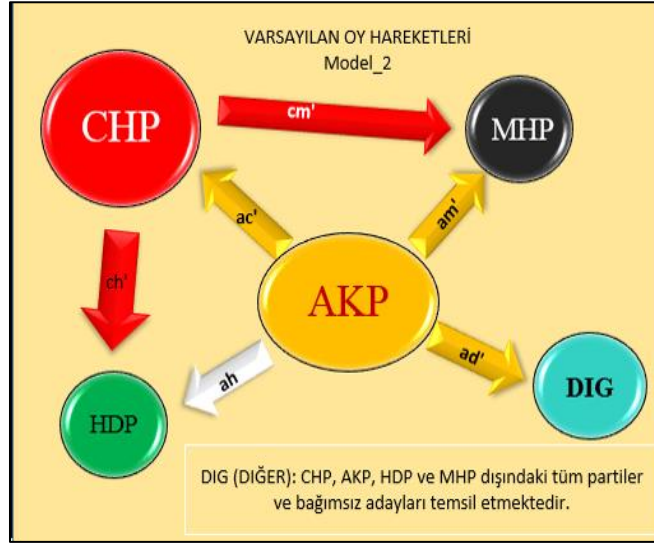
Şekil 2: Model_2 partiler arası oy geçişlerinin hesaplanmasında esas alınan matematik model
