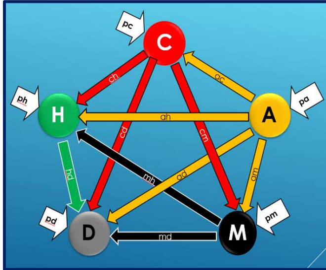
Şekil 1: Partiler arası oy geçişlerinin hesaplanmasında esas alınan matematik model
